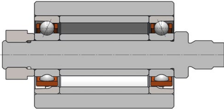
Rigid preload
